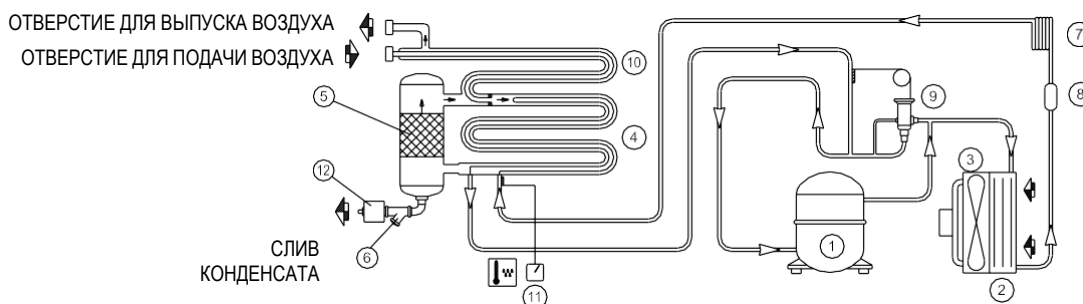
СХЕМА ОСУШИТЕЛЯ
