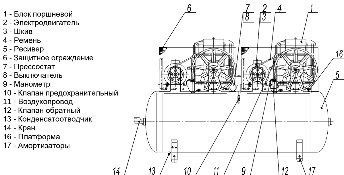
Рисунок 9 - Общий вид компрессора СБ4/Φ-500.AB678TB
