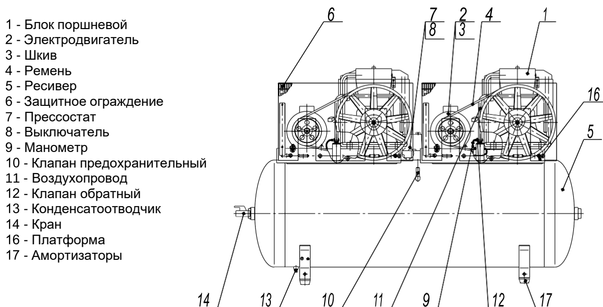
Рисунок 9 - Общий вид компрессора СБ4/Ф-500.AB678ТБ
